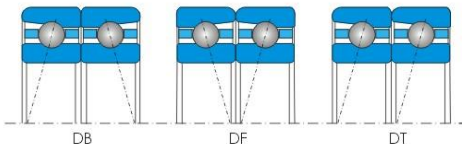
轴承双联配置形式 Duplex Pairings
