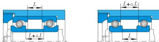
Fig. 13 Position preload
